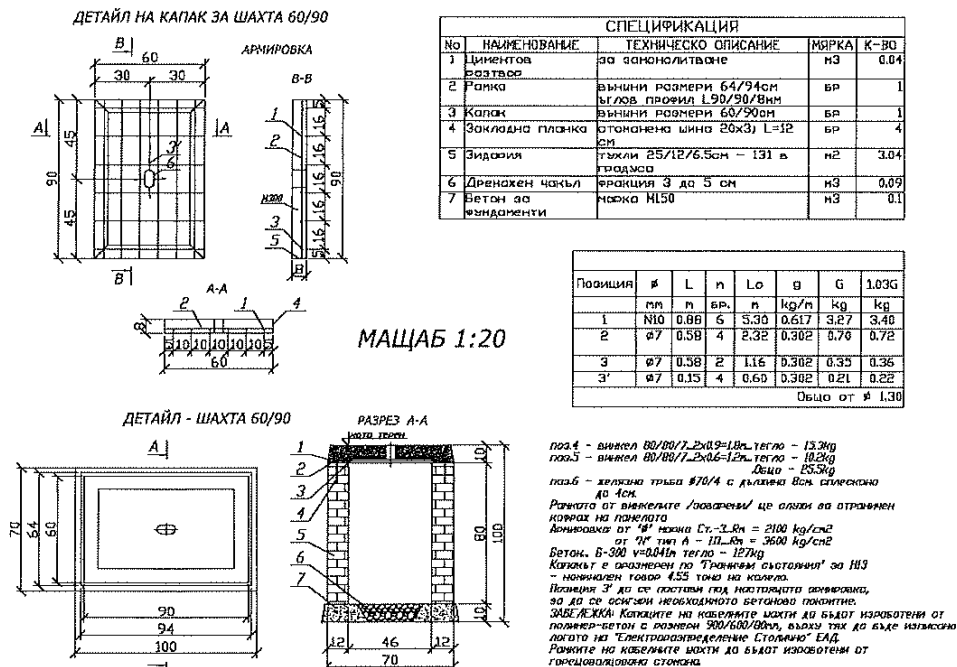
Фиг. 1. Кабелна шахта – единична
